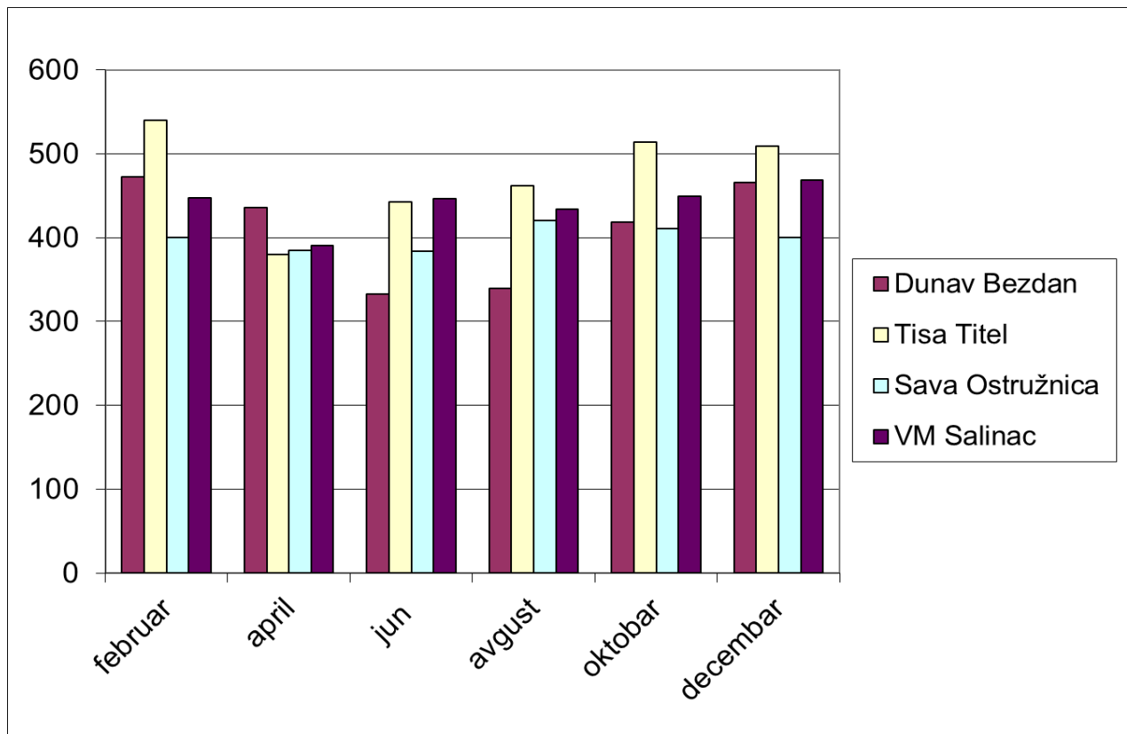
Slika 14. Poređenje vrednosti mesečnih medijana elektroprovodljivosti na Dunavu (prvo merno mesto Bezdán) i poslednjih mernih mesta na pritokama.
