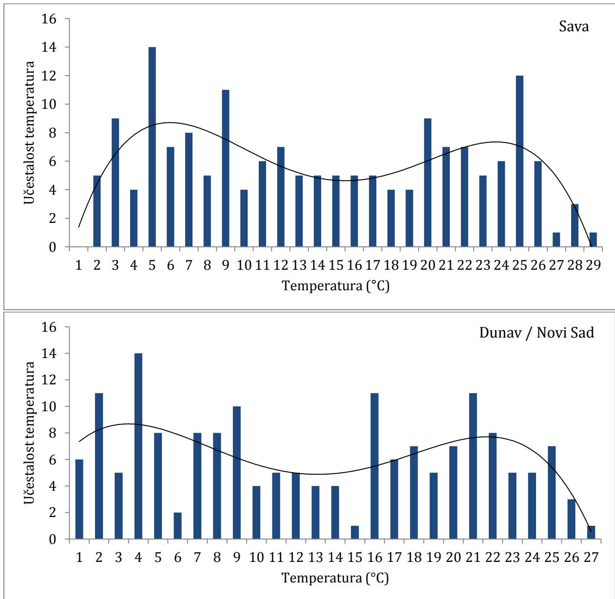
Slika 45. Učestalost javljanja temperatura na poslednjem mernom mestu na Savi (gore) i na mernom mestu Novi Sad (dole). Zavisnost učestalosti od temperature je izražena pomoću polinomijalne funkcije 4. stepena, čiji oblik jasno sugeriše da je raspodela bimodalna.
