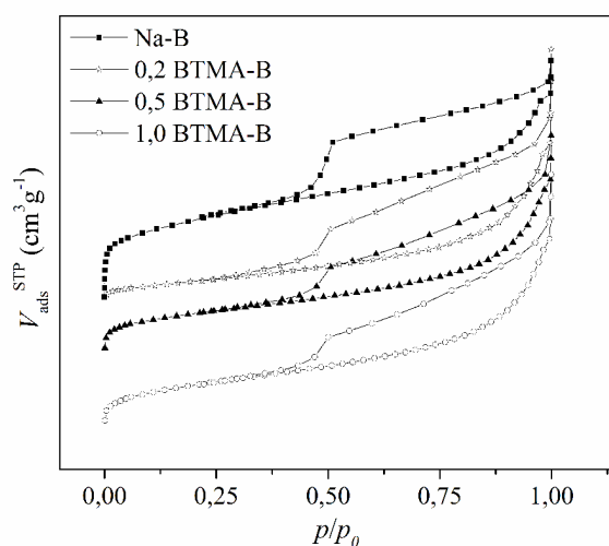
Slika 23. Adsorpciono-desorpcione izoterme azota dobijene za modifikovane uzorke na bazi bentonita iz nalazišta „Bogovina“.
