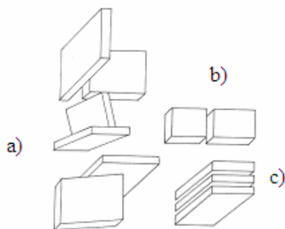
Slika 4. Šematski prikaz slaganja taktoida: a) površina- ivica, b) ivica-ivica, c) površina- površina [30].
