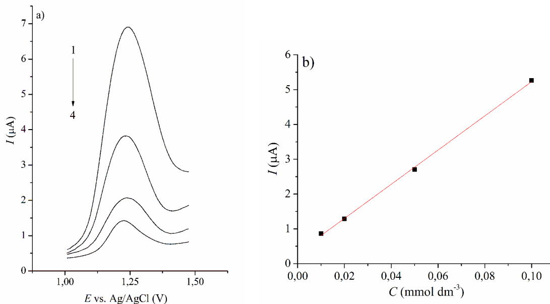
Slika 39. Određivanje 4-nitrofenola DPV metodom pomoću GCE modifikovane sa 1,0 BTMA-B: a) DPV voltamogrami 4-nitrofenola koncentracije: 1) 0,10; 2) 0,05; 3) 0,02 i 4) 0,01 \text{mmol dm}^{-3} i b) odgovarajuća kalibraciona kriva.
