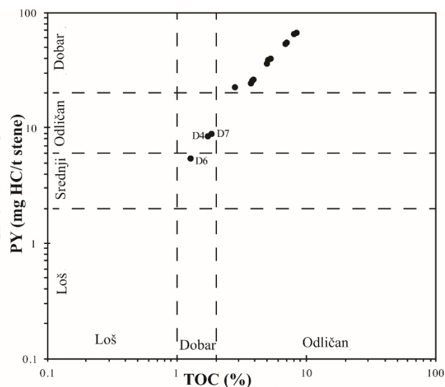
Slika 50. Dijagram PY u zavisnosti od TOC.
