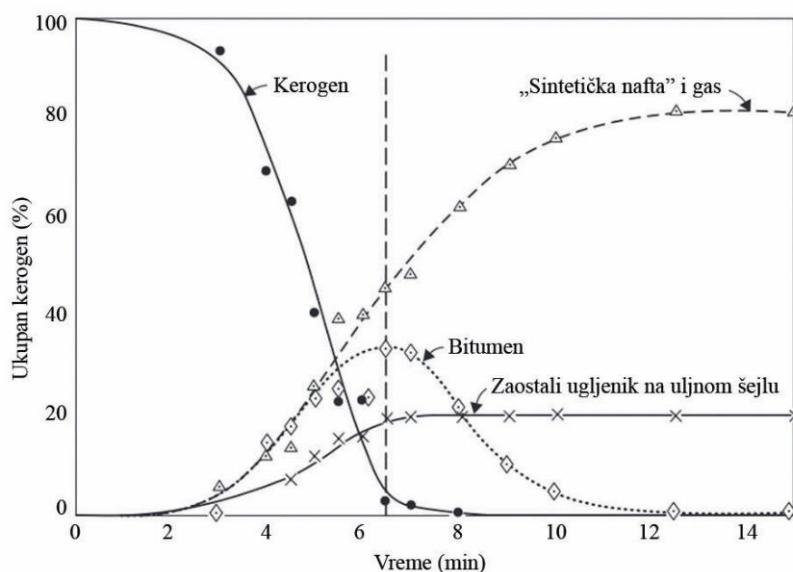
Slika 24. Promene u distribuciji kerogena i proizvoda pirolize tokom vremena (Hubbard & Robinson, 1950).
